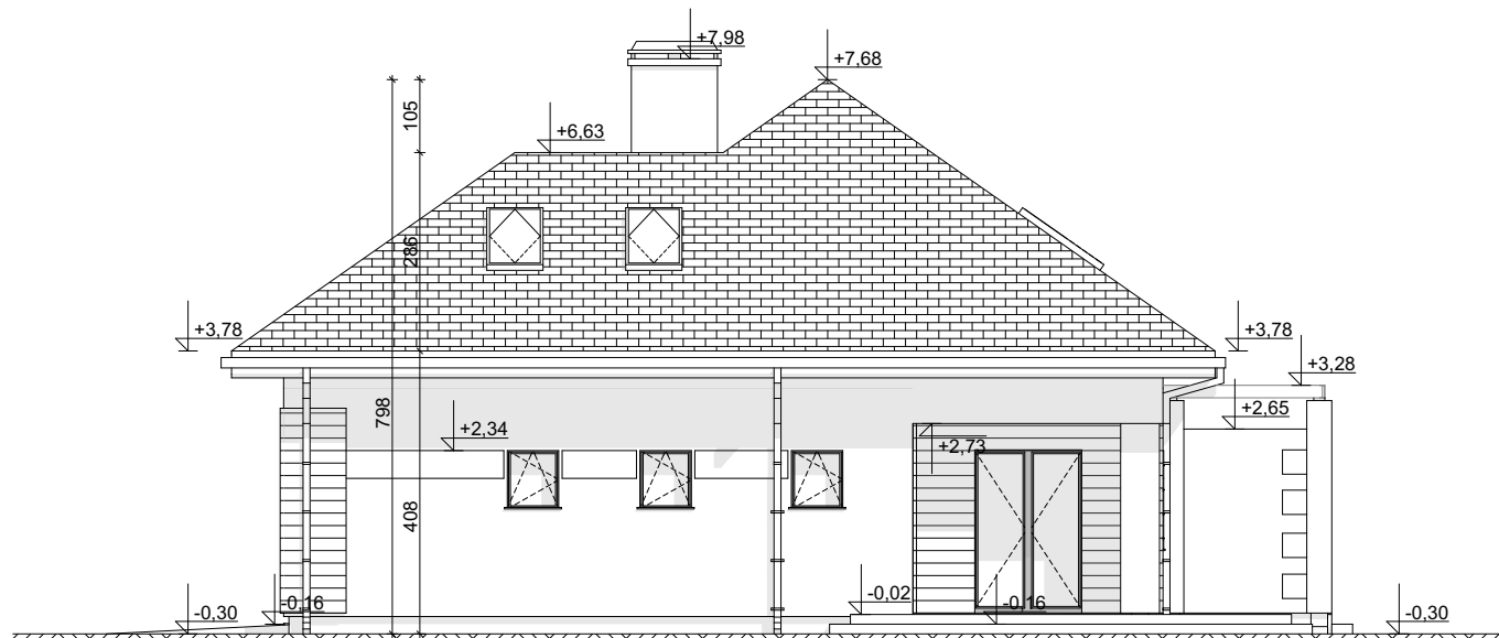
ELEWACJA BOCZNA
