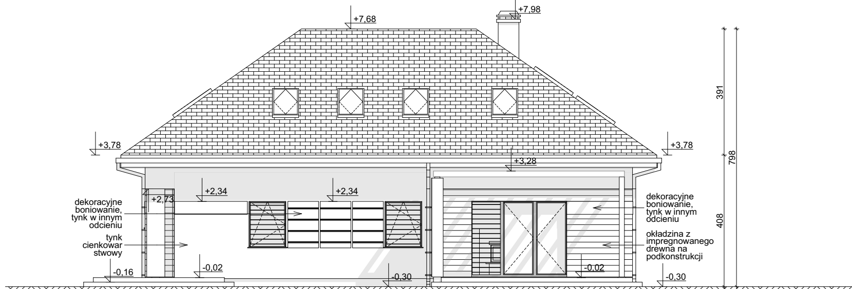
ELEWACJA OGRODOWA
