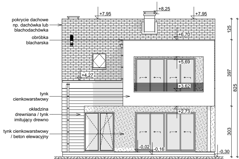
ELEWACJA OGRODOWA
