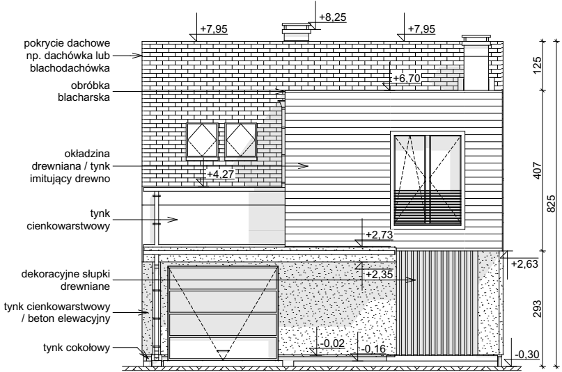
ELEWACJA FRONTOWA
