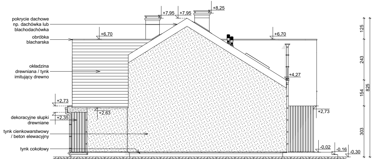
ELEWACJA BOCZNA
