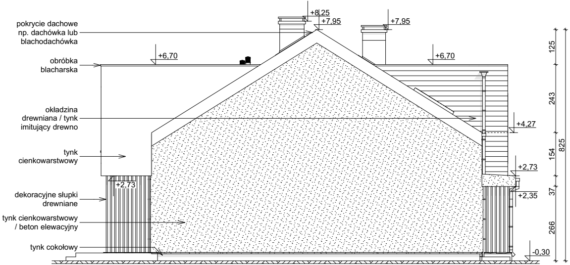
ELEWACJA BOCZNA
