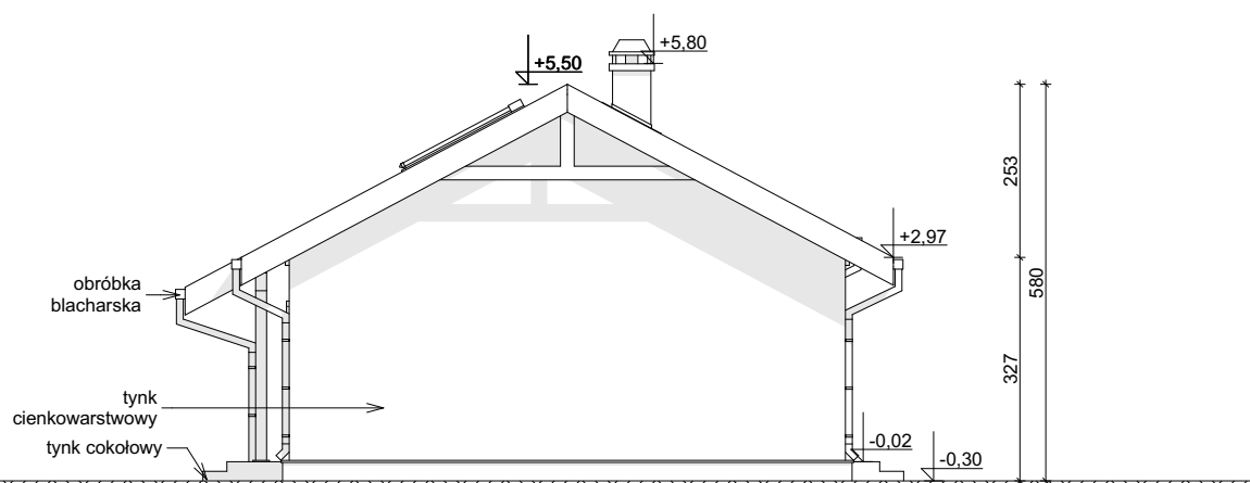
ELEWACJA BOCZNA
