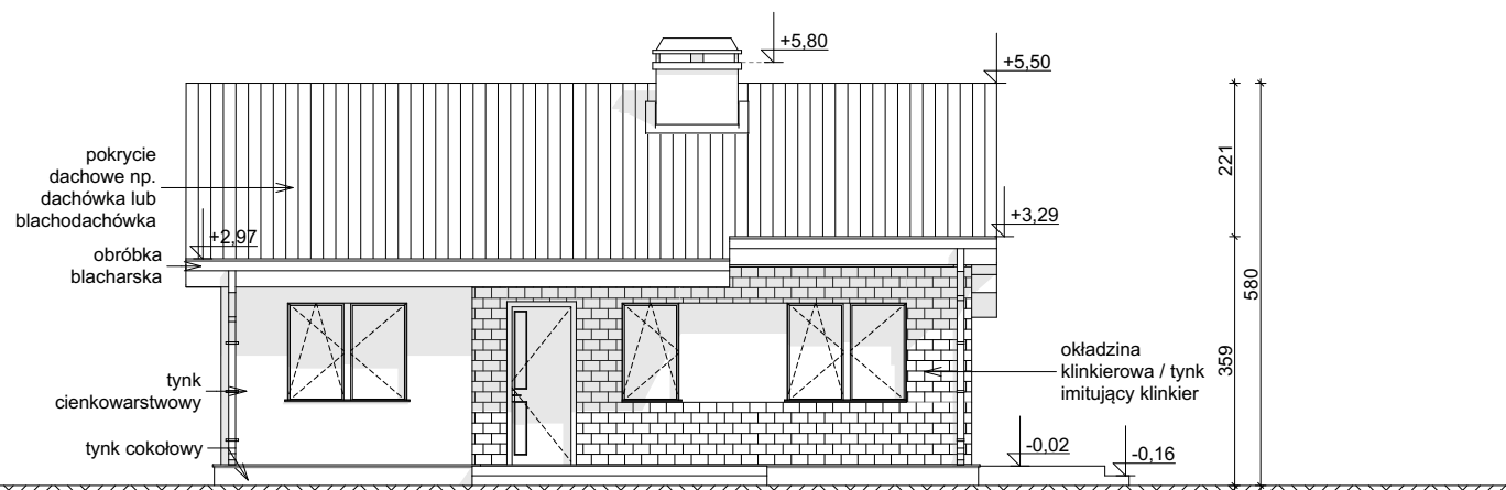
ELEWACJA FRONTOWA
