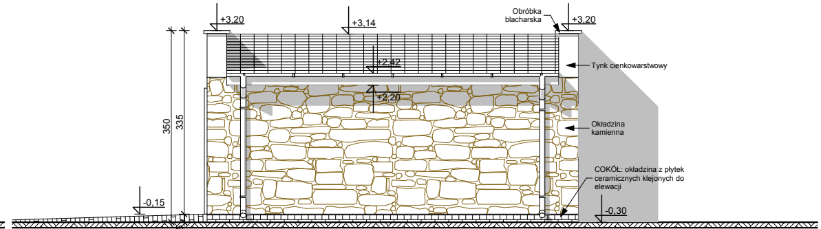
ELEWACJA BOCZNA
