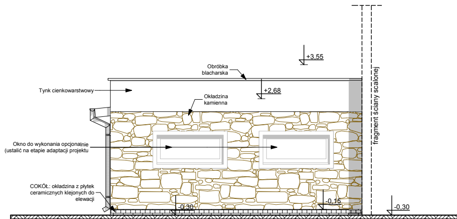
ELEWACJA OGRODOWA
